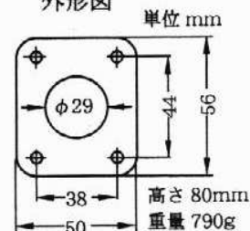
外形図
