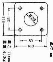
外形図
