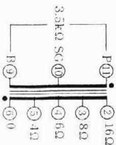
結線図
