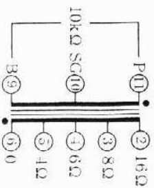
接続図
