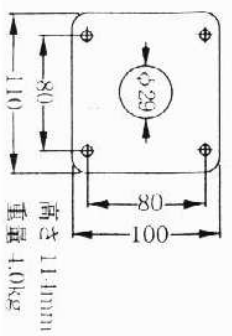
外形図
