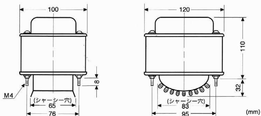
寸法図
