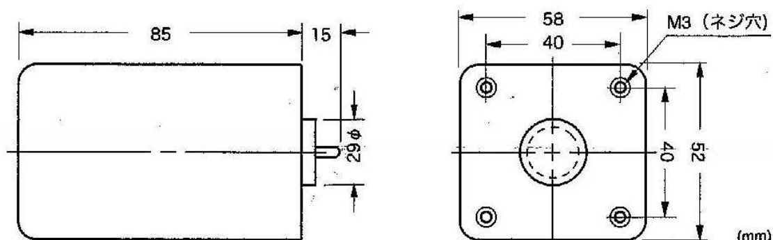
WE - 60 寸法図
